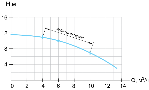
ГНОМ, ГНОМ-LC 6-10
