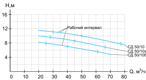
СД 50/10
