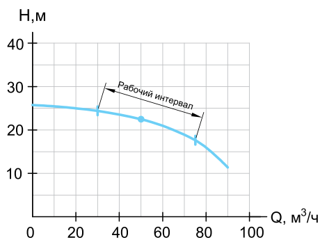
ГНОМ, ГНОМ-LC 50-25
