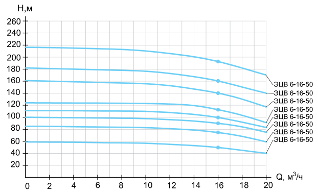
ЭЦВ 6-16
