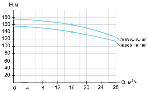
ЭЦВ 8-16
