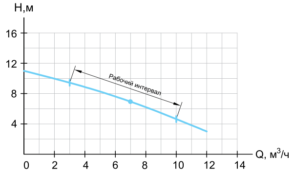
ГНОМ, ГНОМ-LC 7-7
