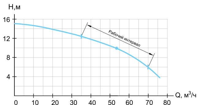
ГНОМ, ГНОМ-LC 53-10
