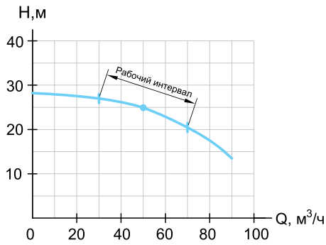
ЦМФ 50-25
