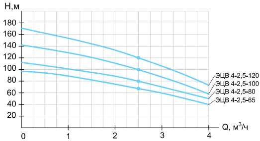
ЭЦВ 4-2,5
