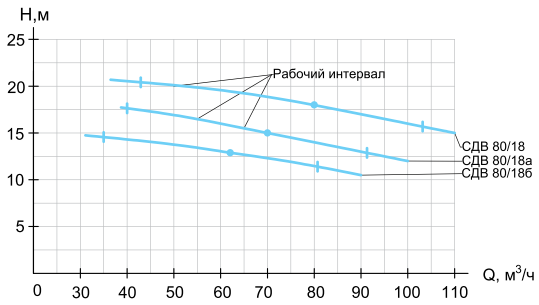
СДВ 80/18
