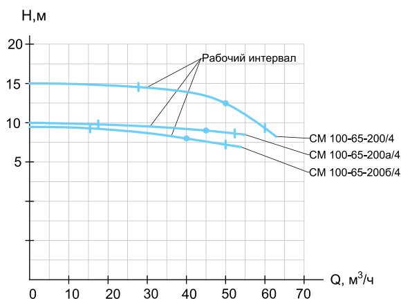
CM 100-65-200/4
