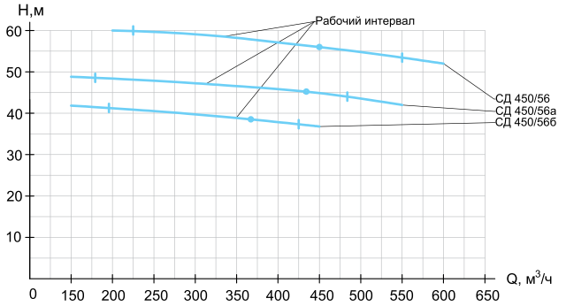
СД 450/56
