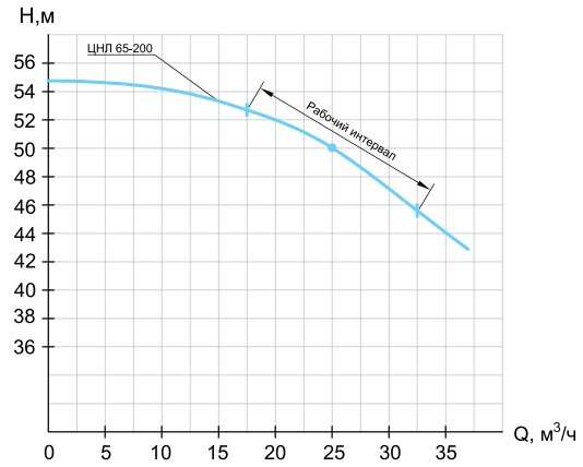
ЦНЛ 65-200
