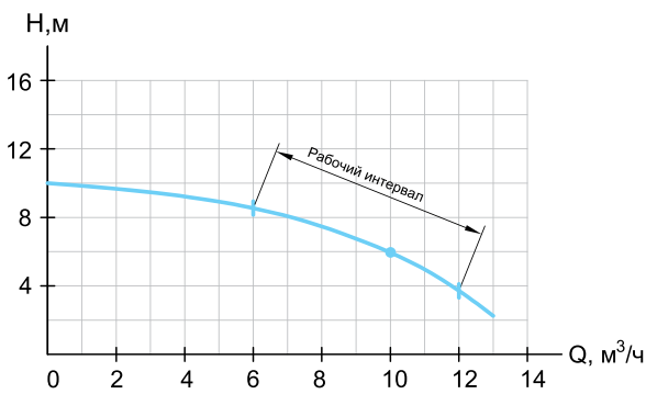
ГНОМ, ГНОМ-LC 10-6
