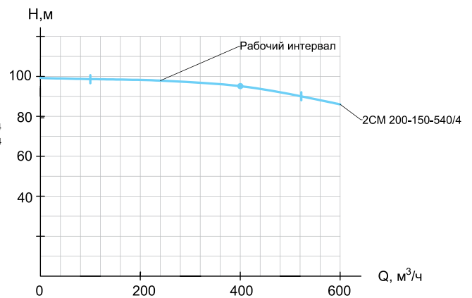
CM, 2CM 200-150-540/4
