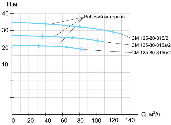
CM 125-80-315/2
