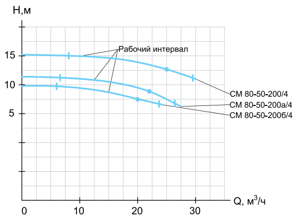
CM 80-50-200/4
