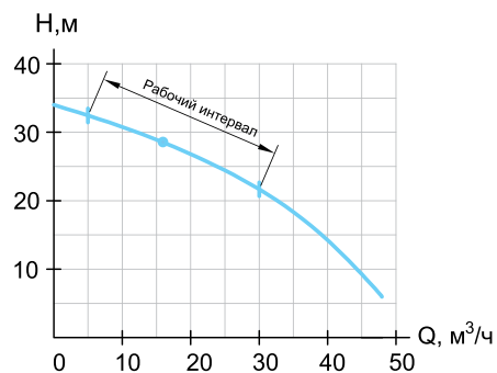
ГНОМ, ГНОМ-LC 16-27
