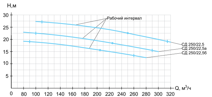
СД 250/22,5
