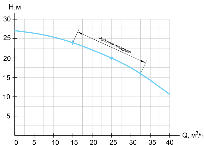
ГНОМ, ГНОМ-LC 25-20
