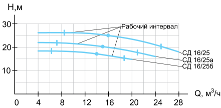
СД 16/25
