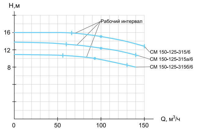
CM 150-125-315/6
