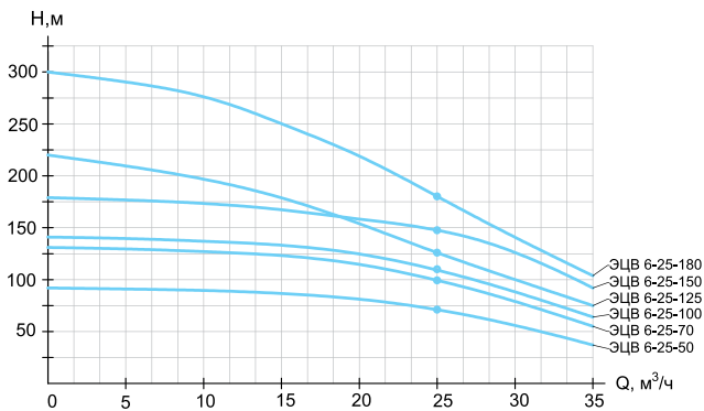
ЭЦВ 6-25
