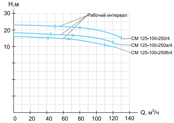
CM 125-100-250/4
