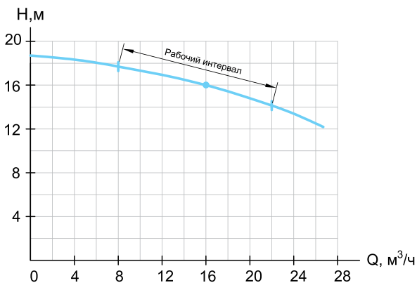
ГНОМ, ГНОМ-LC 16-16
