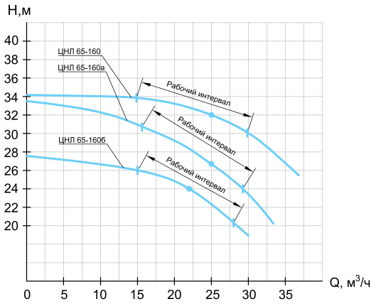
ЦНЛ 65-160
