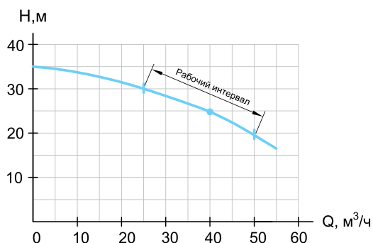
ГНОМ, ГНОМ-LC 40-25
