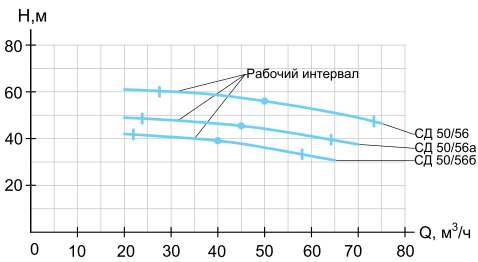
СД 50/56
