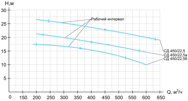
СД 450/22,5
