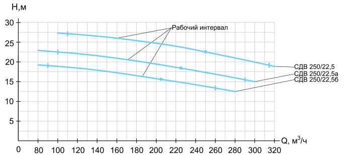
СДВ 250/22,5
