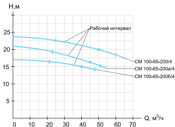
CM 100-65-250/4
