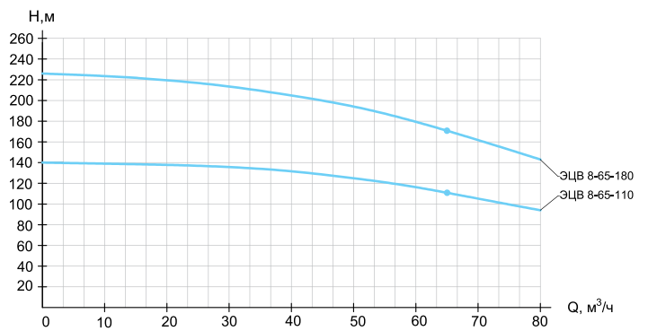
ЭЦВ 8-65
