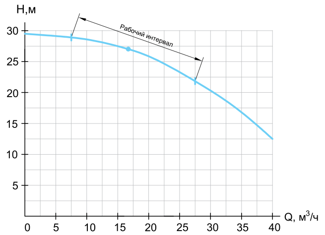
ЦМК 16-27 режущий
