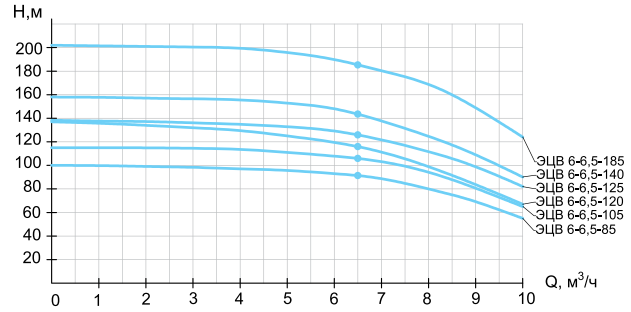
ЭЦВ 6-6,5
