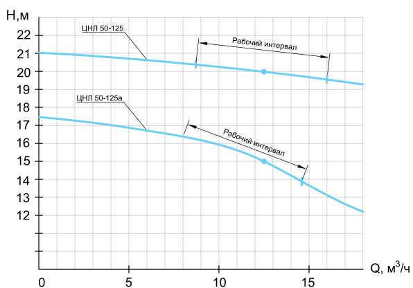
ЦНЛ 50-125
