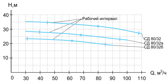
СД 80/32
