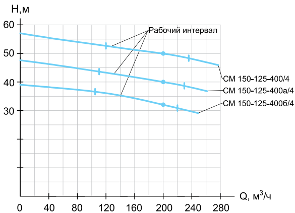
CM 150-125-400/4
