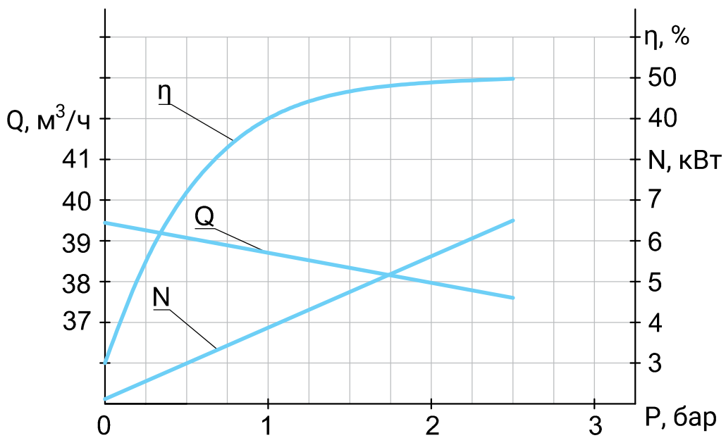
Ш 80-2,5
