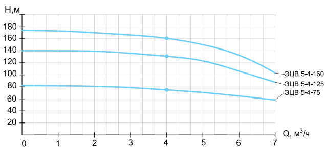
ЭЦВ 5-4
