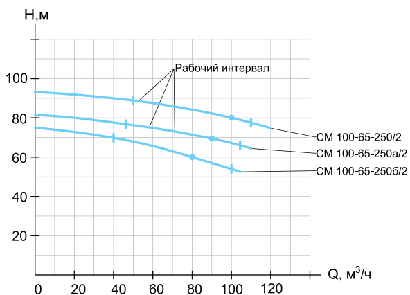
CM 100-65-250/2
