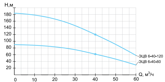
ЭЦВ 6-40
