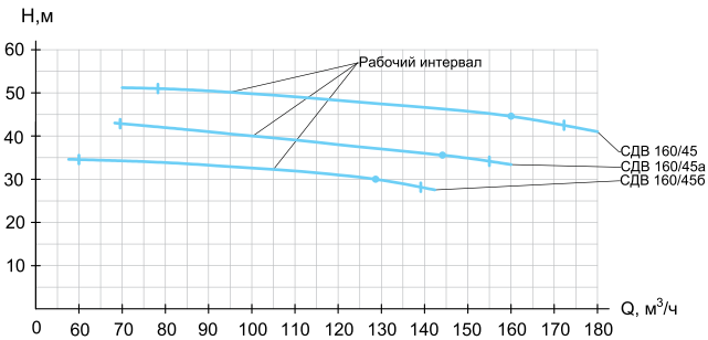
СДВ 160/45
