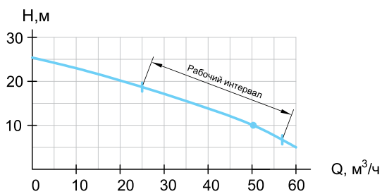
ЦМФ 50-10 режущий
