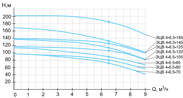
ЭЦВ 4-6,5
