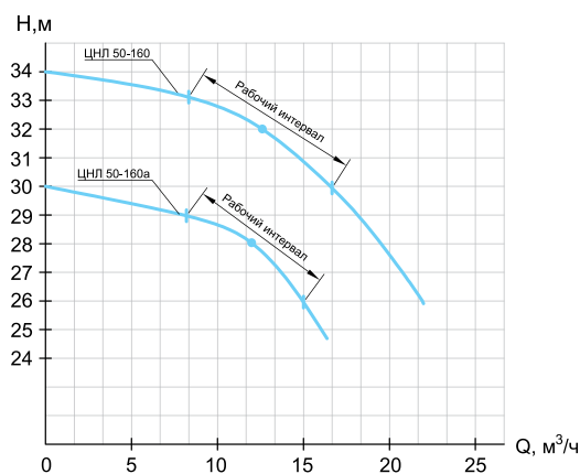
ЦНЛ 50-160
