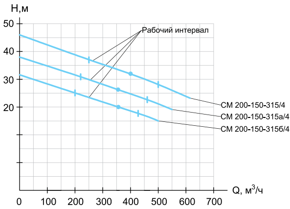
CM 200-150-315/4
