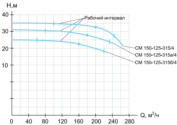
CM 150-125-315/4
