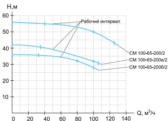
CM 100-65-200/2
