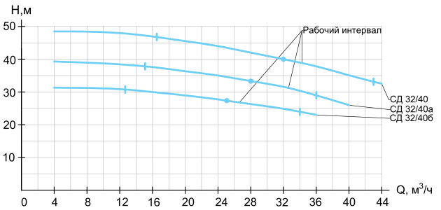
СД 32/40
